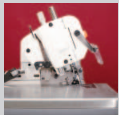
Kettentrenner seitlich Side chain cutter
