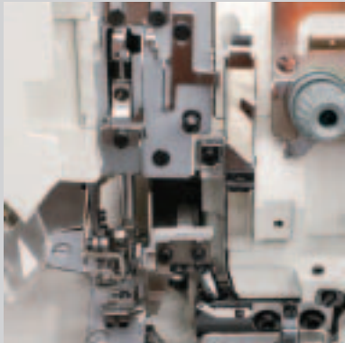
Nadel- und Fadenschmierung Needle and thread lubrication
